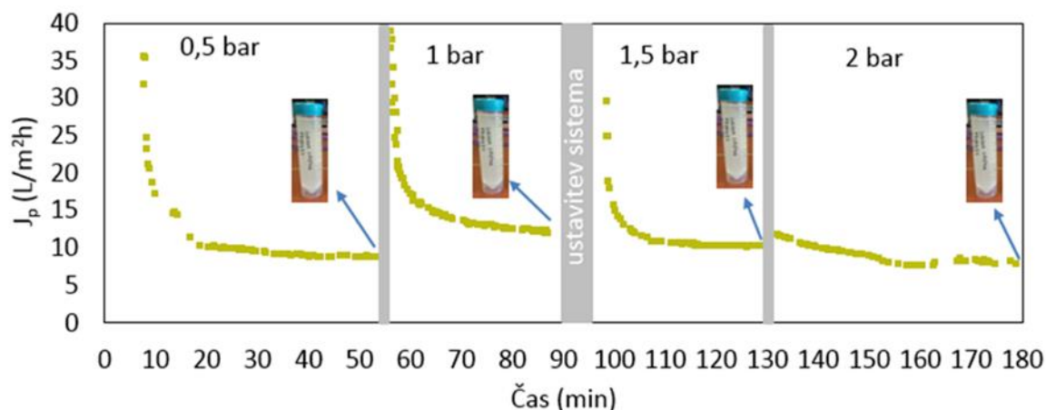
Slika 1: Pretok sirotke pri različnih tlakih.
