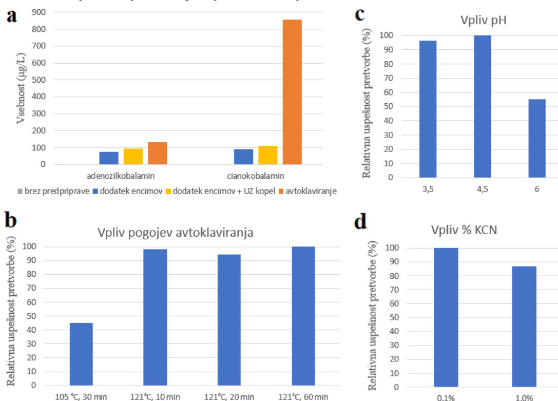
Slika 1: Vpliv dejavnikov na nastanek CNCbl; a – vpliv metod za razbitje bakterijskih celic na sprostitve vitamina B 12 , b – vpliv pogojev avtoklaviranja, c – vpliv pH raztopine s KCN, d – vpliv % KCN. Relativno uspešnost pretvorbe (%) smo podali glede na najboljši rezultat.
