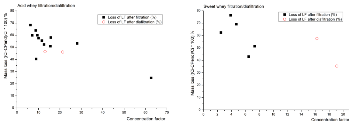
Slika 2: Masne izgube LF tekom filtracije/diafiltracije glede na vhodno maso LF v sirotki v odvisnosti od koncentracijskega faktorja filtracije in tipa filtracijskega procesa.
