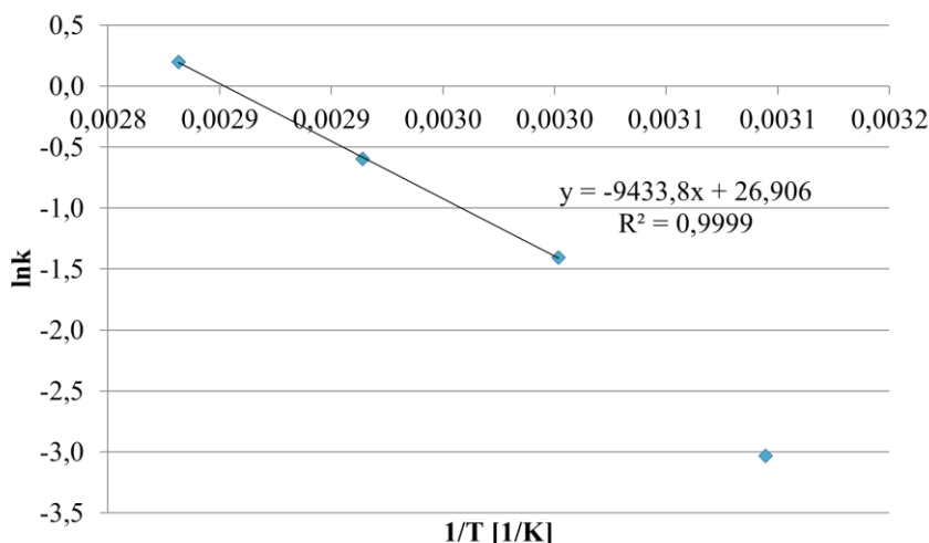
Slika 1: Arrheniusov graf za vzorec izolata Lf 1 ( c = 1.0 \text{ mg/mL} ), ki temelji na konstantah hitrosti razpada 0. reda za razpad Lf med 50 in 80 °C.
